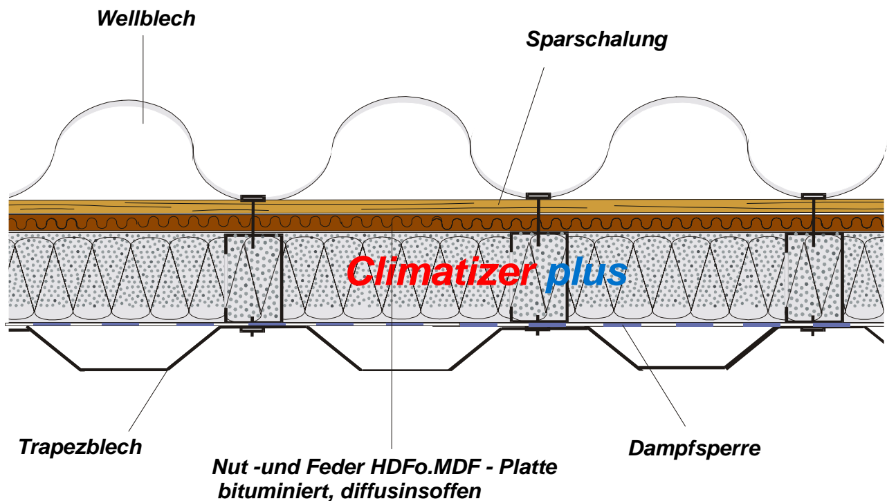
Detail I1
